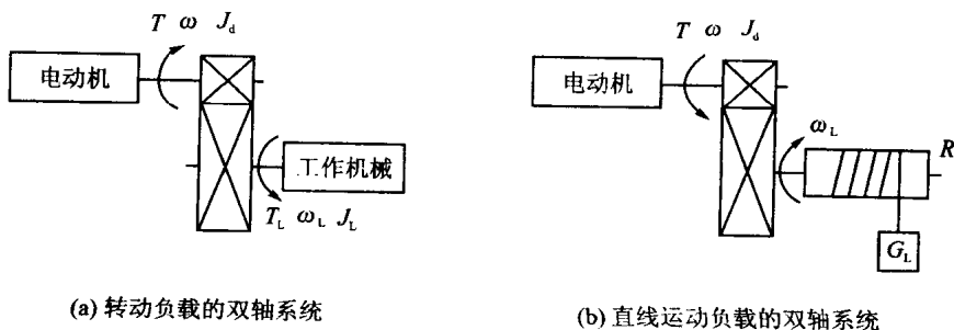
图 1-3 双轴传动系统
