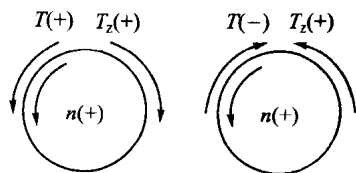
图 1-2 转矩方向符号约定
