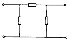
图 1-4 \pi 形网络
