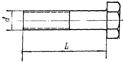
GB 5-76 六角头螺栓(粗制)图
