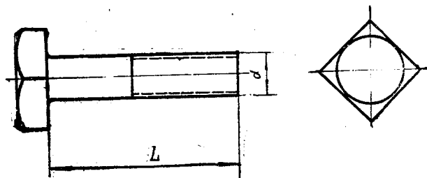
GB 8-76 方头螺柱图 (粗制)
