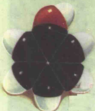
苯酚
