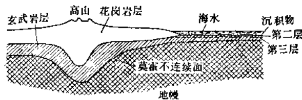
图 1-4 地壳构造断面图
