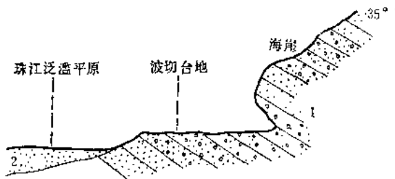
图 1-7 广州七星岗波切台、海岸剖面图 1—第三纪红色砂岩、砾岩；2—现代冲积层
