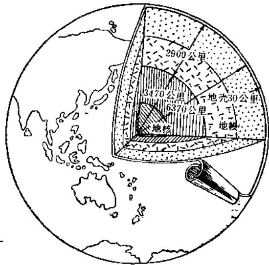
图 1-3 地球构造示意图
