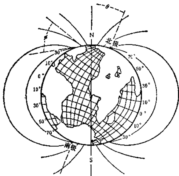
图 1-6 地磁要素及地球周围磁力线分布示意图 \theta —磁偏角； \phi —磁倾角
