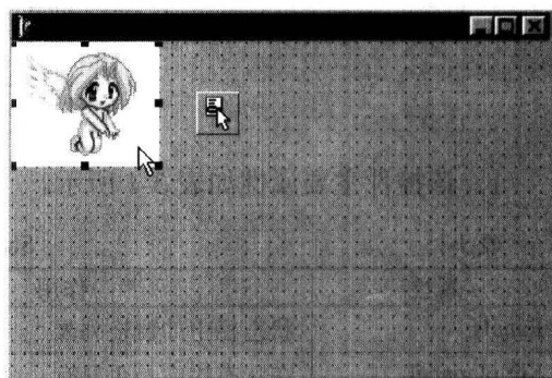
图 2-4 设计期界面
