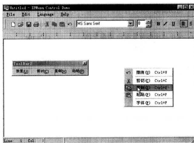
图 1-2 运行界面图 (2)
