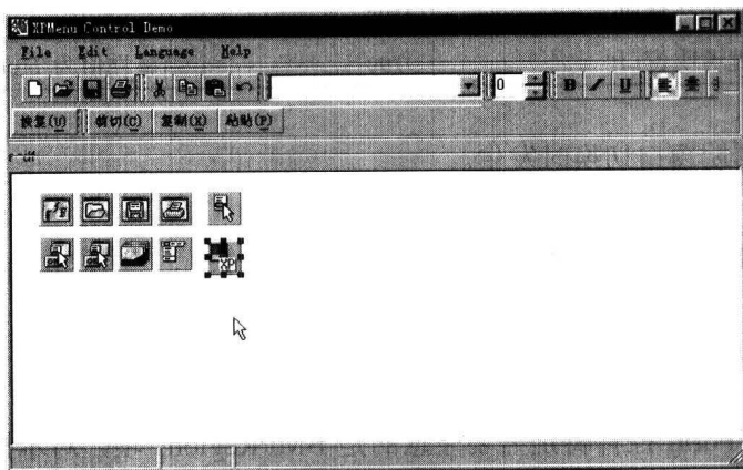
图 1-5 设计期界面
