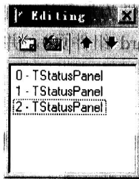
图 3-3 窗格编辑器
