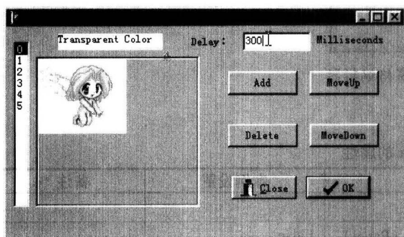
图 2-3 属性编辑
