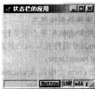
图 3-2 运行界面图 (2)
