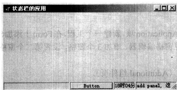
图 3-1 运行界面图 (1)
