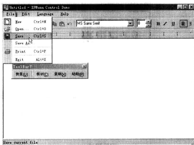
图 1-1 运行界面图 (1)
