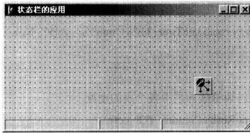
图 3-4 设计期界面
