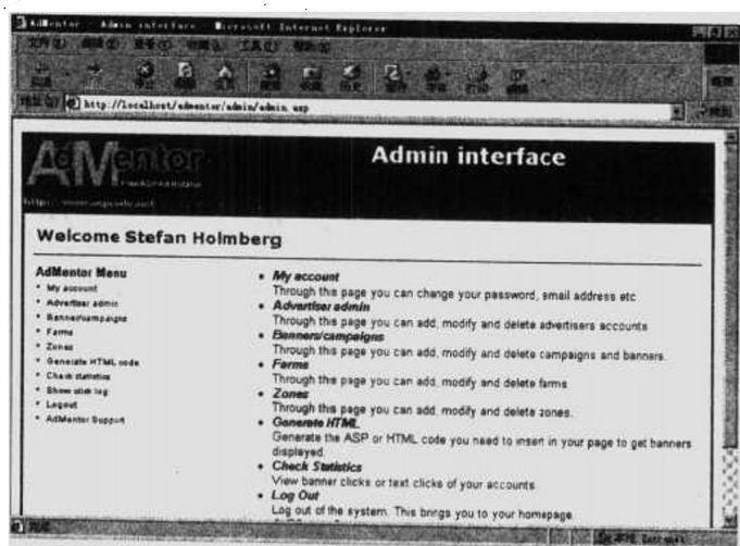
图 1.7 程序 4 的界面
