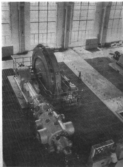
尿素设备之一——二 氧化碳压缩机
