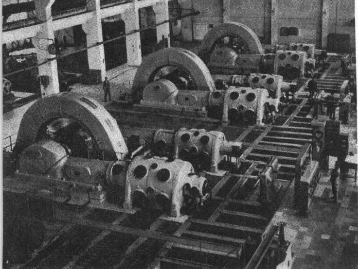
合成氨车间一角——高压压缩机
