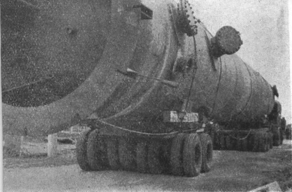
身重近百吨的水洗 塔躺在三十六个轮胎 的平板运输汽车上
