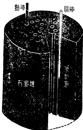
圖1 反应堆当中的石墨堆示意图。实物当中共有152条孔道，每条孔道有1条鈾棒或鎳棒。
