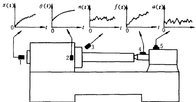
图2 某机床工作状态监测系统
