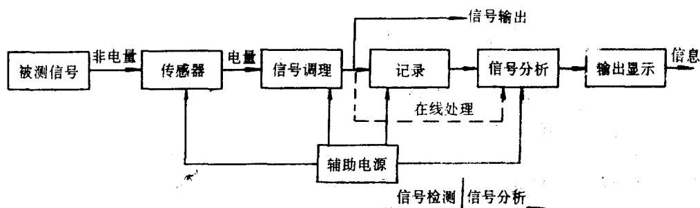
图 3 典型电测方法的测量过程
