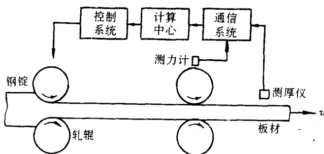
图1 自动化轧钢系统
