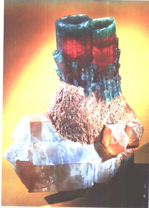
电气石
