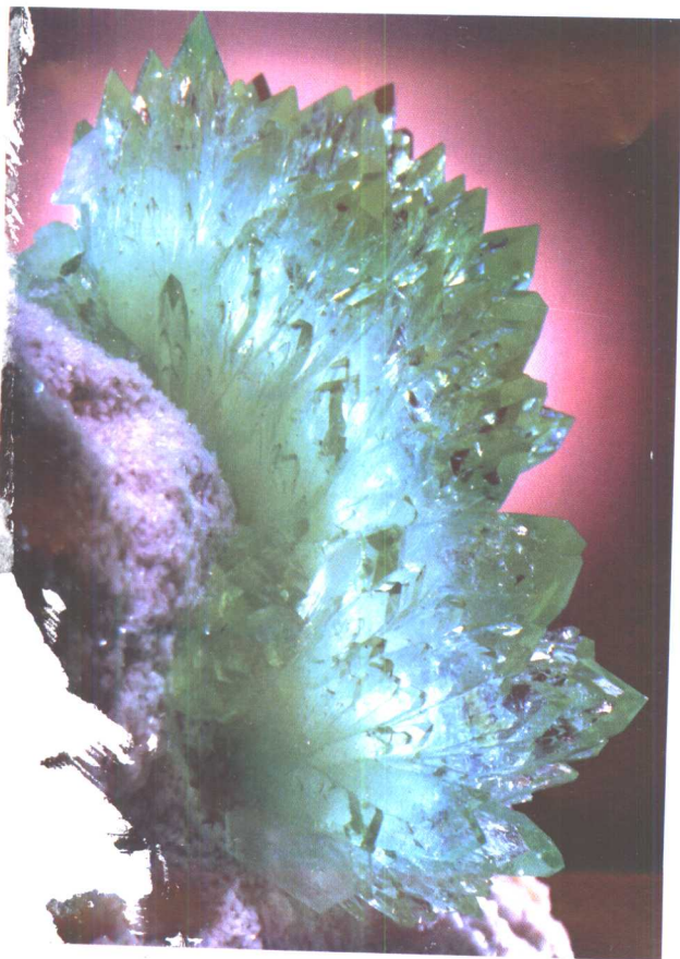
鱼眼石
