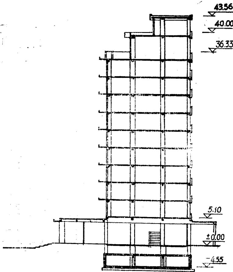
图 3 剖面图
