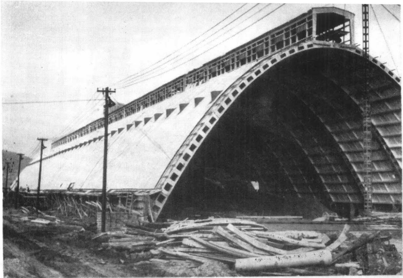
班斯卡—比斯特立查煉鋁工廠的新創造—— 新式的弓形水泥倉庫
