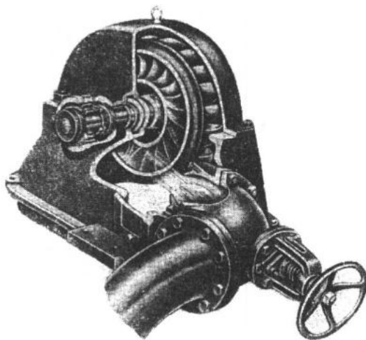
图 1-10 斜击式水轮机
