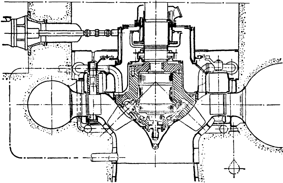
图 1-4 XL003-LJ-160 斜流式水轮机剖面图
