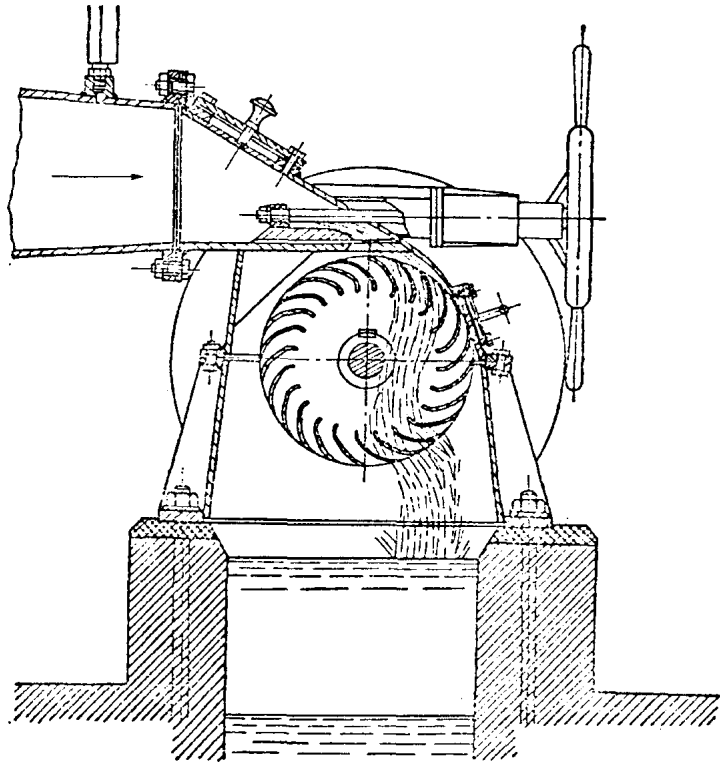
图 1-11 双击式水轮机
