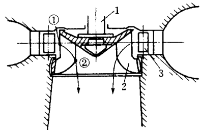
图 1-2 混流式水轮机
