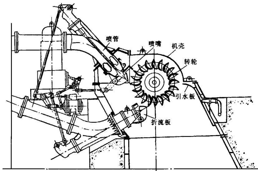
图 1-9 水斗式水轮机
