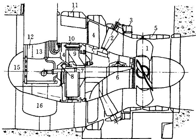
图 1-8 灯泡贯流机组
