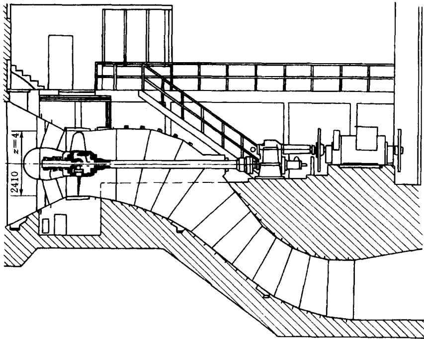
图 1-6 轴伸贯流式机组
