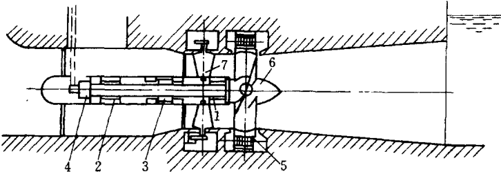
图 1-5 全贯流式水轮机
