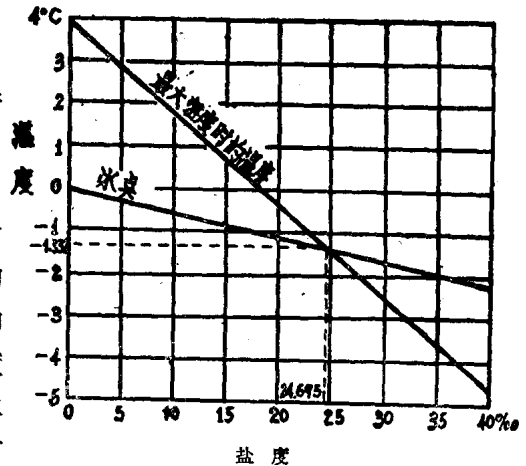
图1—3 含盐量对水溶液凝结温度及最大密度时温度的影响
