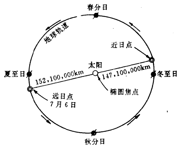
图 1.1.4 地球公转运动 地轴与黄道面法线有 23.5^\circ 度夹角
