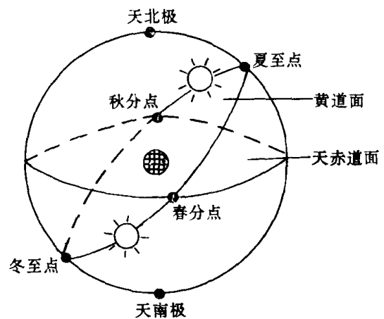
图 1.1.6 天球坐标系
