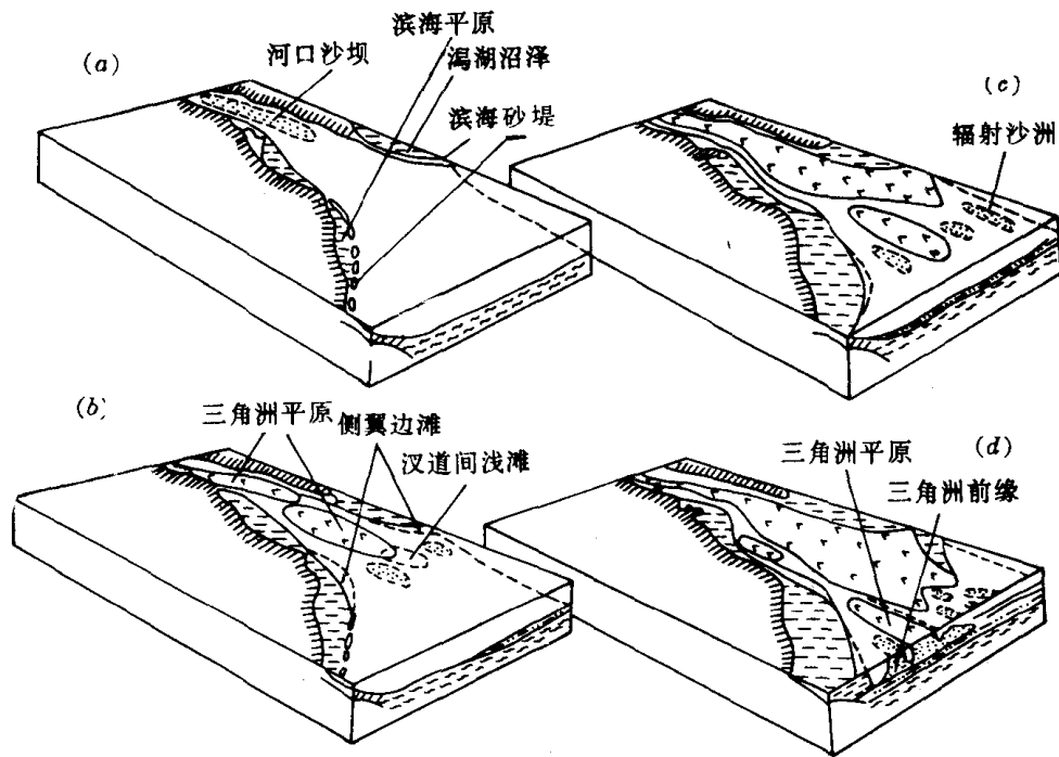
从 a d. 长江口左岸不断发育沙洲、沙坝，由于河道右偏，北支水道不断淤塞，沙坝（岛）并岸，使三角洲不断得到发展
