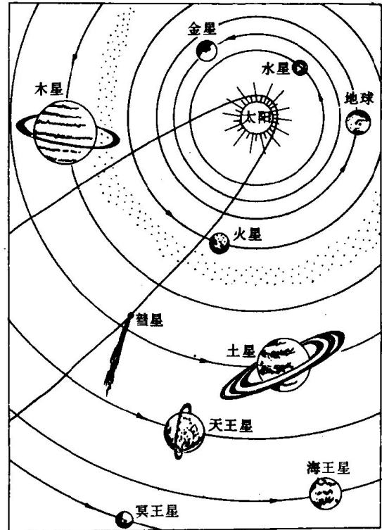
图 1.1.2 太阳系
