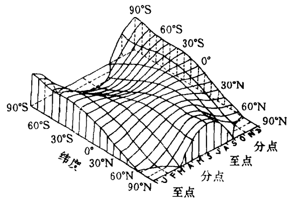
图 1.1.5 不同纬度的全年日照 (取自 Strahlers, 1974)
