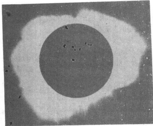
图 1.1.1 我们的太阳 日全食时日冕的形状十分不规则 (Hal Observatory)
