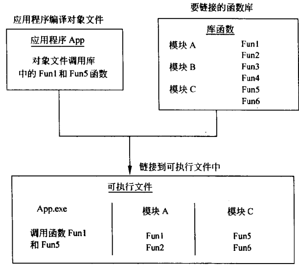
图 1.1 静态链接
