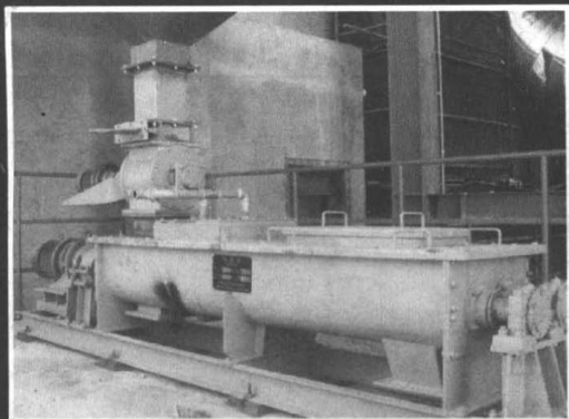
● 双轴加湿机
