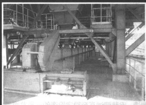
● 刮板输送机
