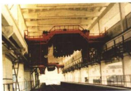
6614A型桥式螺旋卸车机 6614A-type Bridge Screw Unloader
