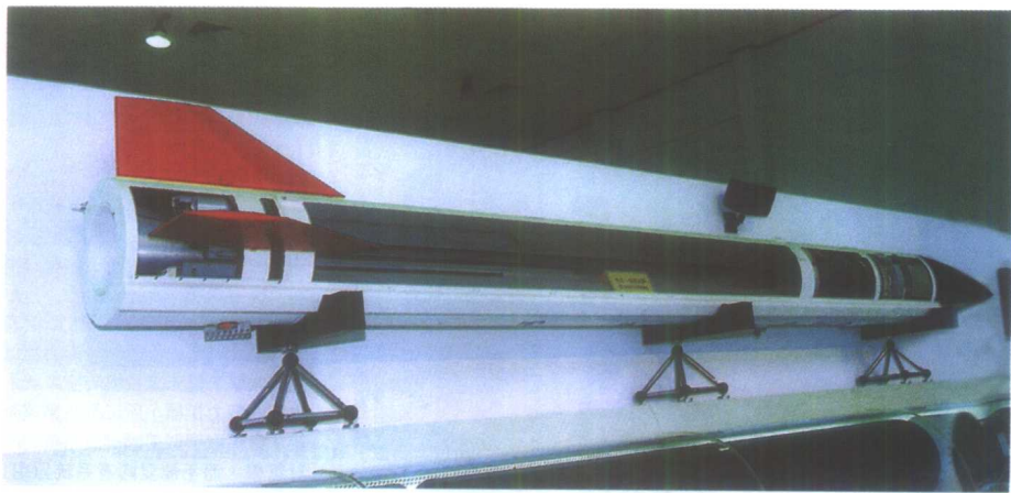
台军“天弓一型”导弹剖面结构
