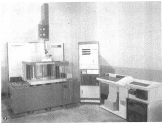
图0-6 三坐标仪——从模型或实物获得数控加工程序,再通过数控程序的几何数据生成零件图纸
