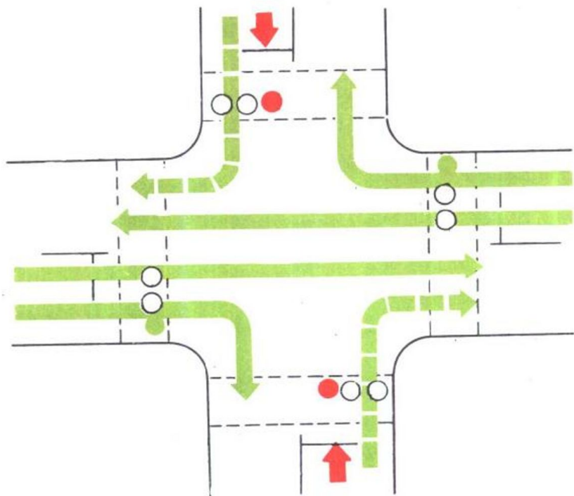
图 1 绿灯亮信号
