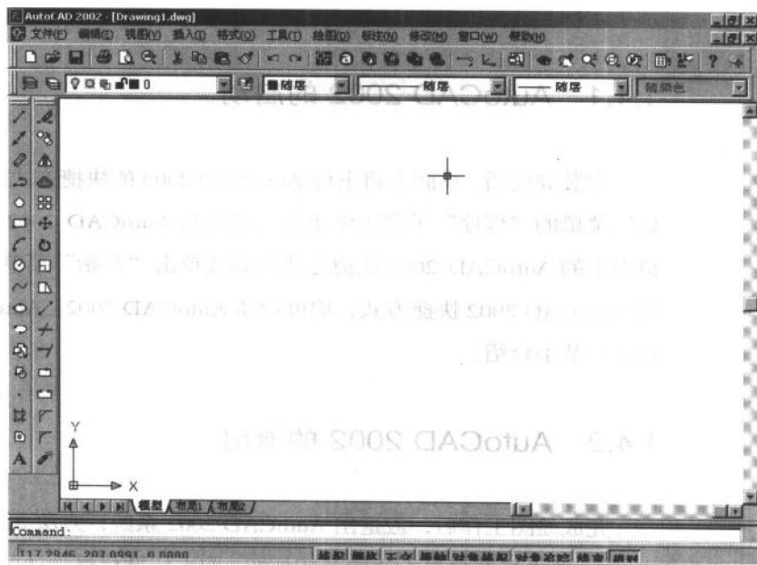
图 1-2 AutoCAD 2002 界面
