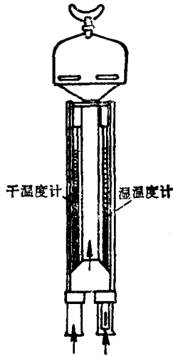
图 1—4 吸风式干湿温度计
