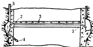
图 1—6 井筒聚水圈
