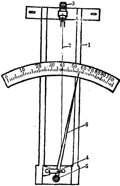
图 1—2 毛发湿度计
