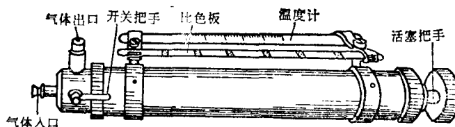
图 1—1 抽气唧筒
