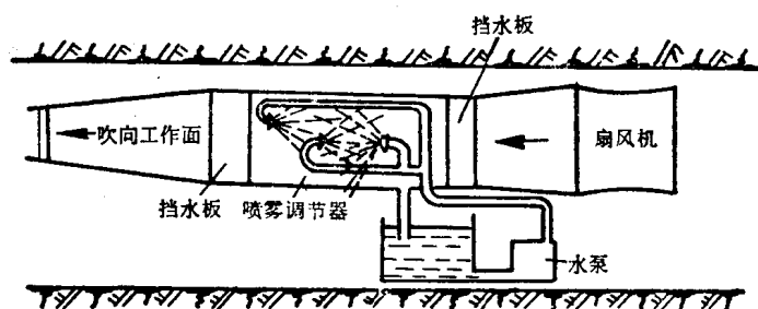
图 1—5 井下降温的喷雾风扇
