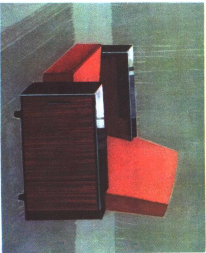
高靠背沙发 总高1000~1020,座 垫前沿距地380,后沿距地320,长 560,宽520,沙发总宽820(连左右 扶手箱计内),扶手箱宽150。座垫与 靠背夹角106°。扶手箱外侧有门,可 将烟酒糖茶,杯碗什物等置于其内。
