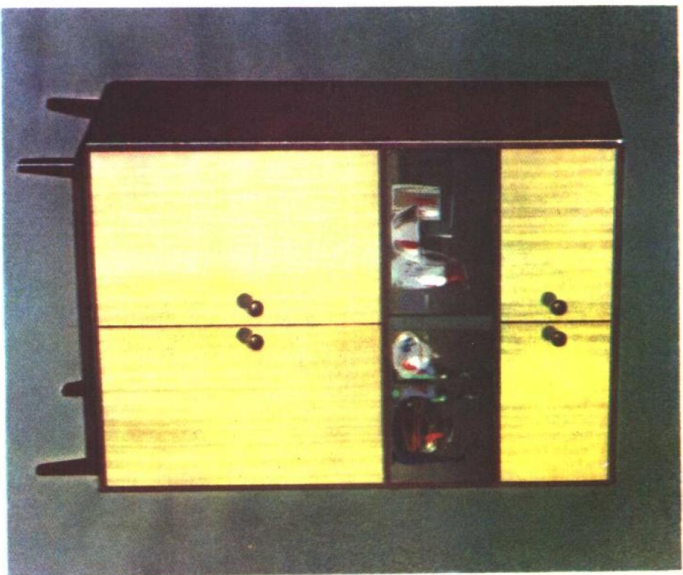
杂物柜 高1800, 宽1100, 厚450。大柜门里有一层搁板。
