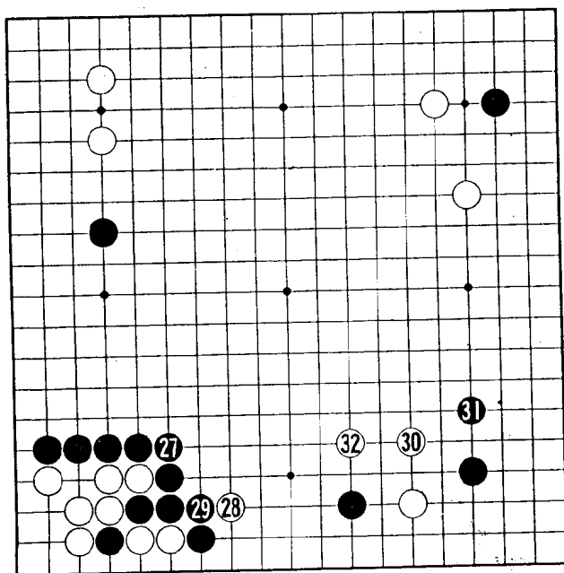
第5谱 (27~32)
