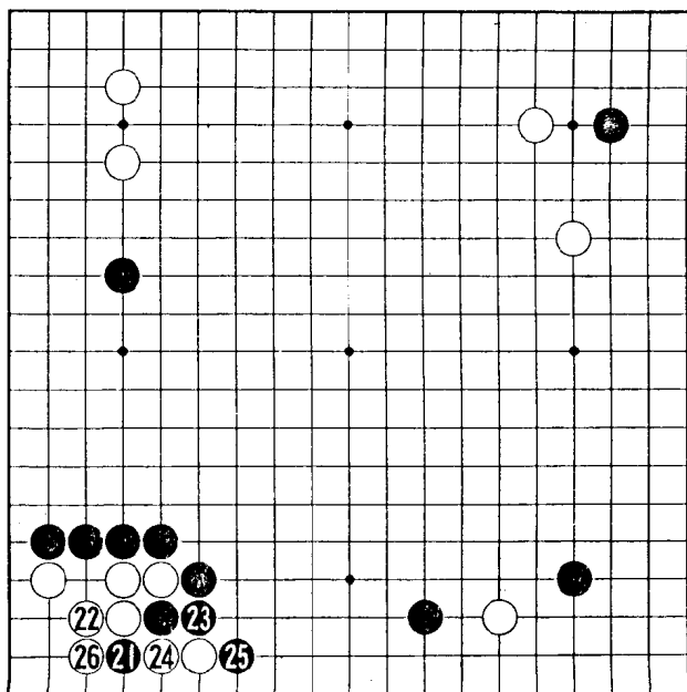
第4谱 (21~26)
