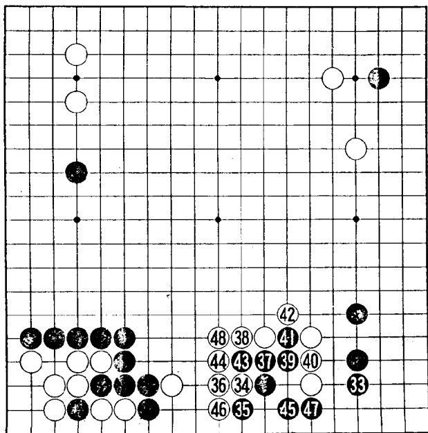
第6谱 (33~48)
