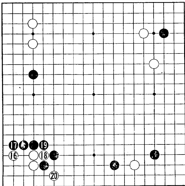
第3谱 (16~20)
