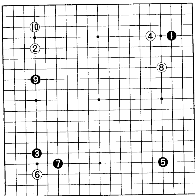
第 1 谱 (1 ~ 10)
