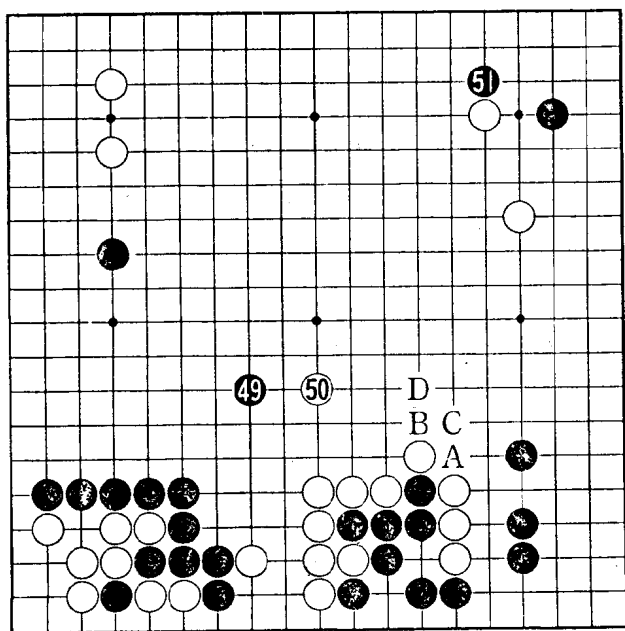
第7谱 (49~51)
