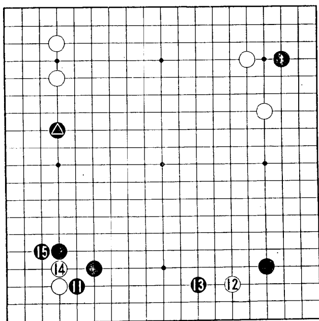
第2谱 (11~15)
