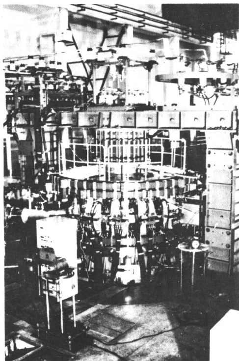
图 9 “中国环流器一号”主机
