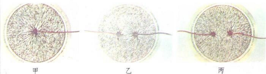
图 1 点电荷的电场
