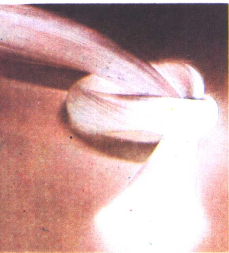
图 5 云室中 \alpha 粒子的径迹 ▶
