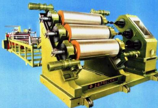
QDYG \phi 400 \times 1400斜式三辊压光机组
