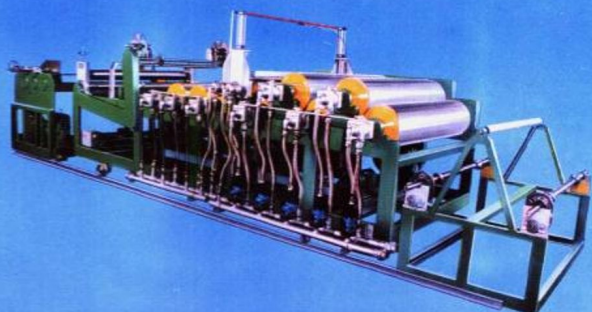
LS1400.PVC热收缩包装膜机组
