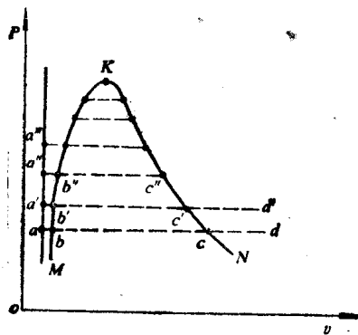
图 2-1 水蒸气的 P - v 图
