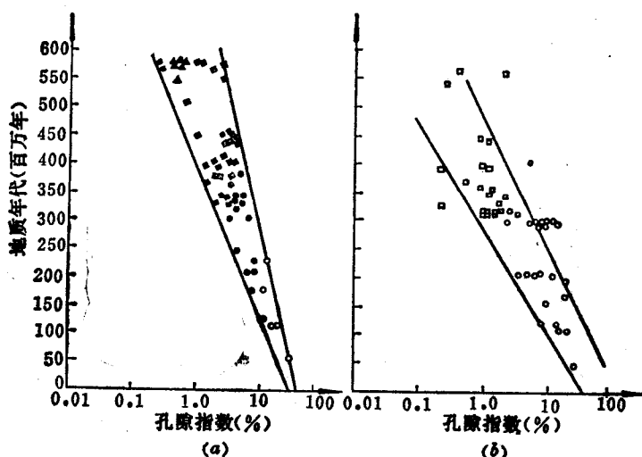
图 2-3 岩石的孔隙指数与地质年代的关系
