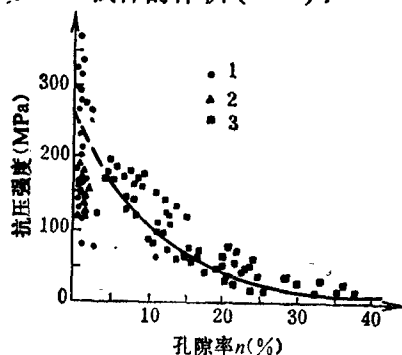
图 2-2 碳酸盐类岩石的抗压强度与孔隙率之关系
