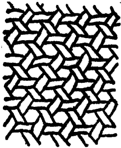
三向平纹结构的织物示意图
