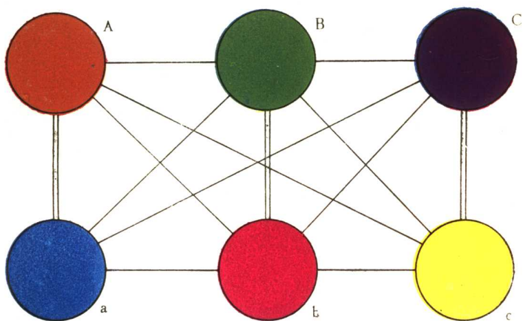
图5-10 光的三原色(A,B,C)与物体的三原色(a,b,c)
