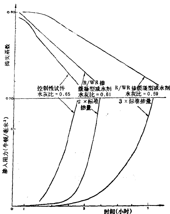
图1-2 缓凝型减水剂对保持工作度的效果
