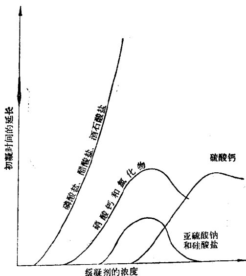
图1-1 各种外加剂对初凝时间的影响
