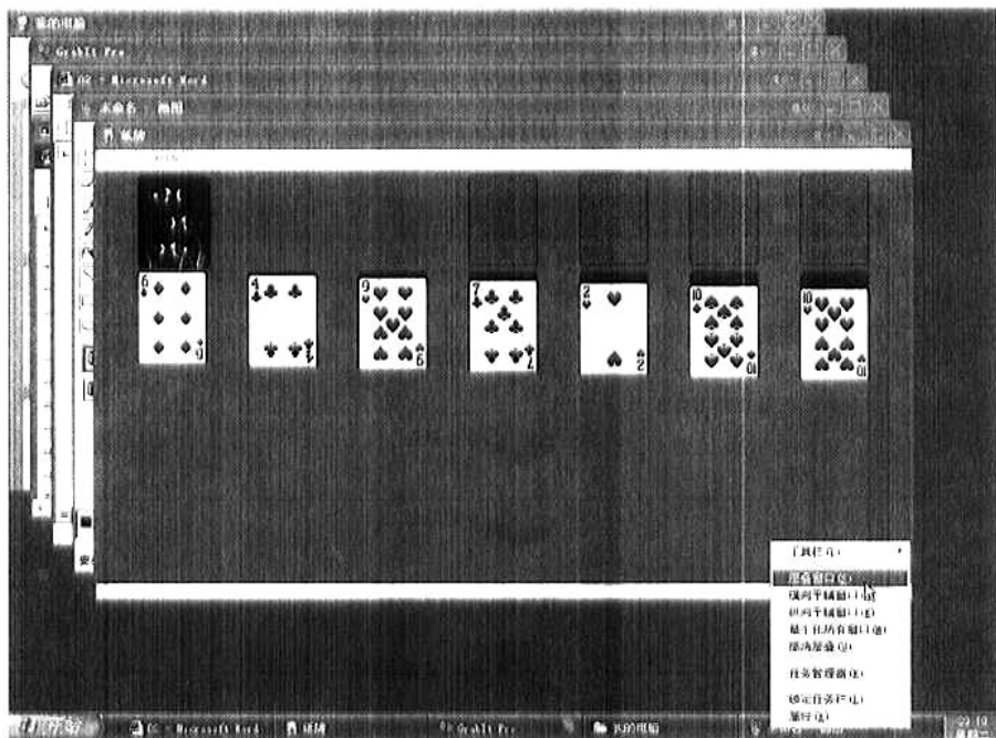
图2-8 层叠窗口
