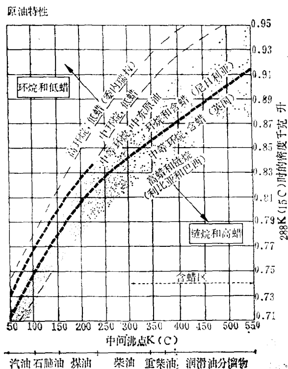
图2.1 各种原油的密度/中间沸点比较
