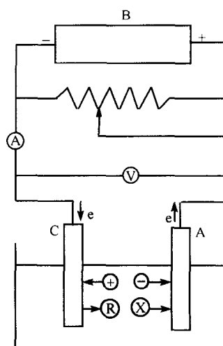
图 1.1 电化学合成系统示意图
