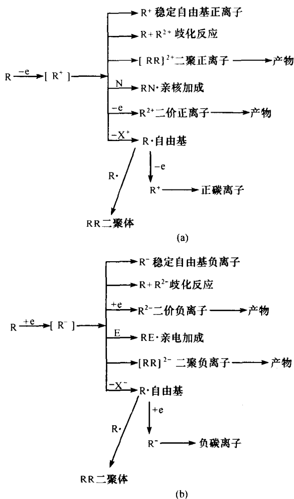
图 1.2 有机电化学合成反应的基本类型
