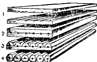
圖4. 你瞧，怎樣從杉松板得出鉛筆來：1，在兩塊木板上都做出凹槽來；2，把石墨條放到凹槽裏，把兩塊木板黏合起來；3，第一次鉋削以後，出現了鉛筆的上面一半；4，第二次鉋削以後，木板變成了六支鉛筆
