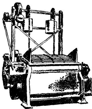
圖3. 混和石墨和膠水的攪拌機
