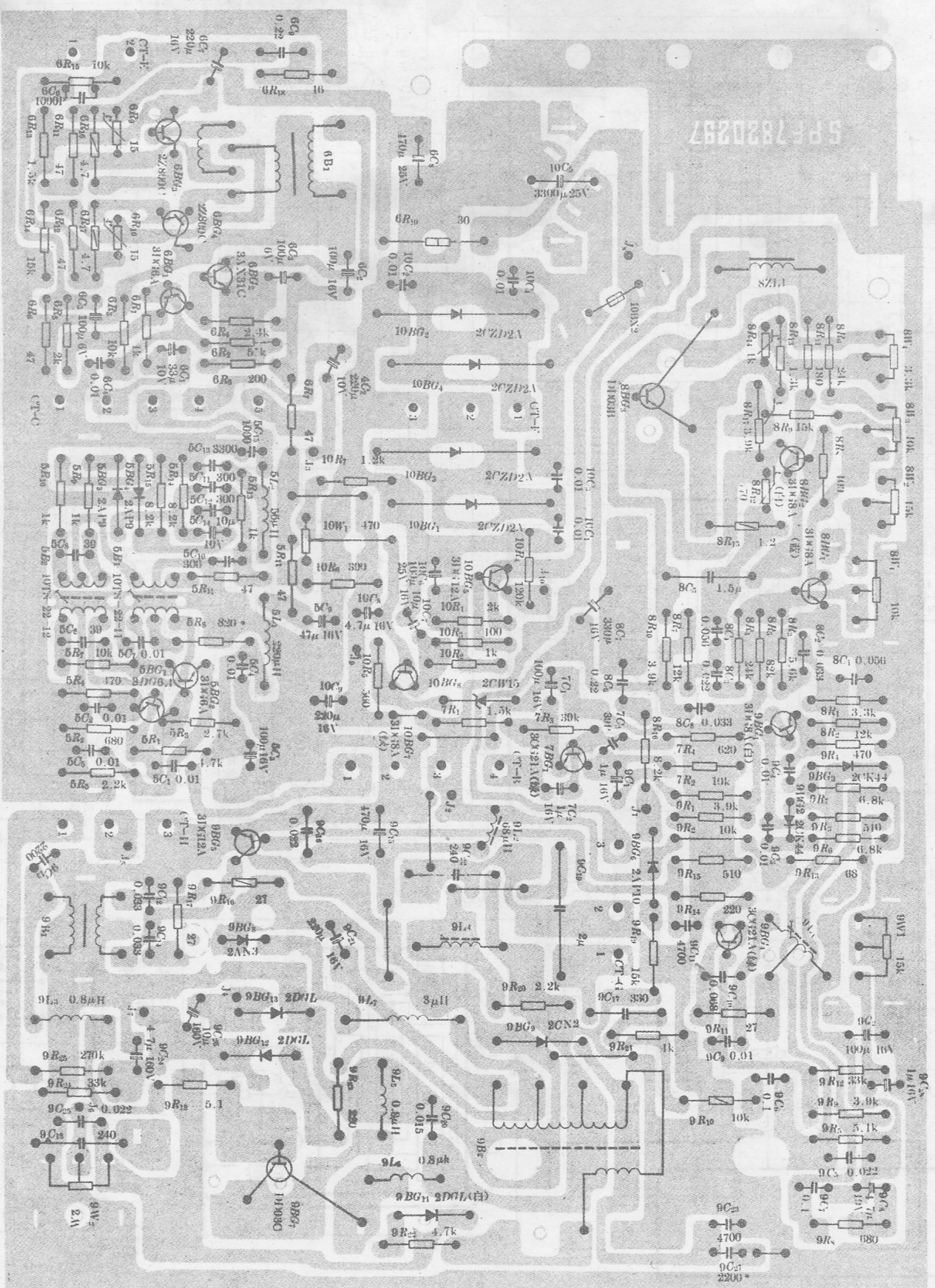
扫描、伴音、电源印制电路板
