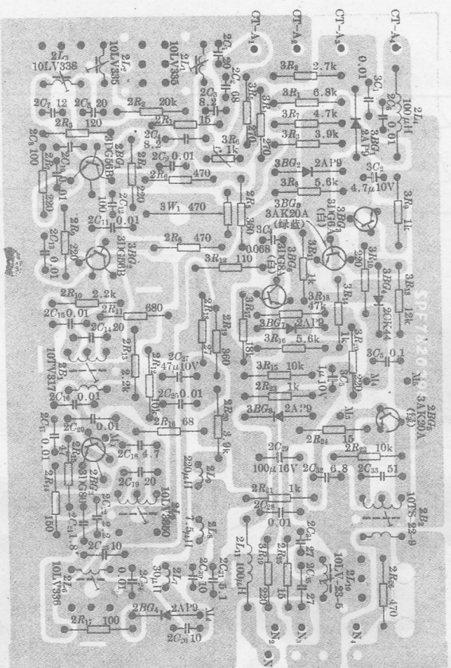
通道印制电路板
