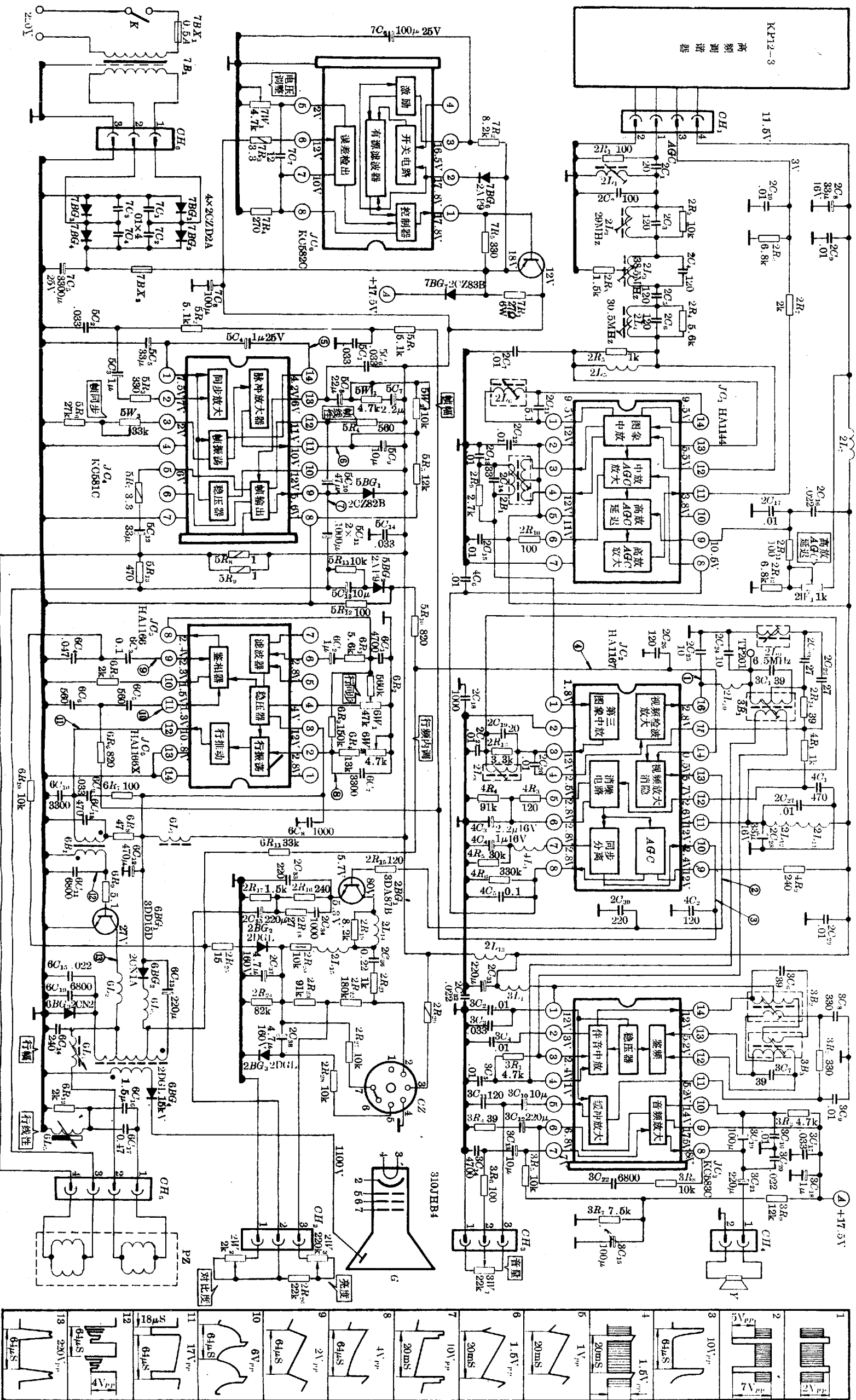
电原理图
