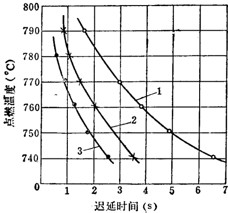
图 3-1-6 温度与点火迟延的关系 1—740℃；2—750℃；3—780℃
