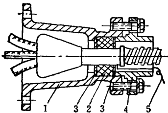
图 3-3-5 铠装电缆进线装置
