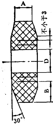
图 3-3-1 橡胶密封垫
