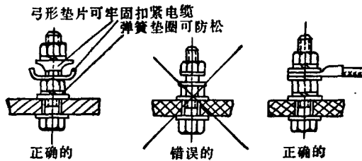
图 3-3-8 导体连接示意图
