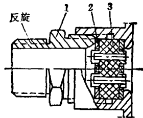
图 3-3-6 钢管布线进线装置
