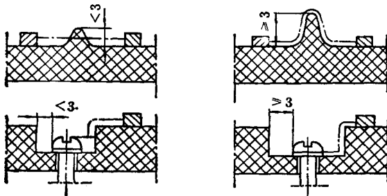
图 3-3-7 漏电距离计算示意图
