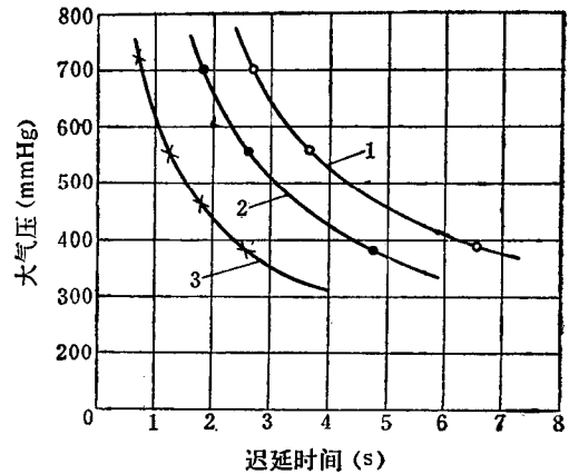
图 3-1-7 压力与点火迟延的关系 1—394mmHg；2—550mmHg；3—704mmHg
