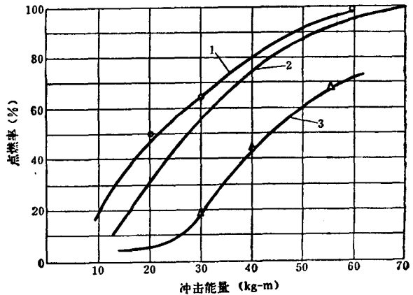
图 3-1-3 冲击能量与点燃或燃率的关系 1—相对湿度90%；2—相对湿度57%；3—干燥状态
