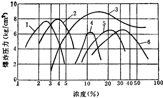
图 3-1-10 爆炸压力与浓度的关系
