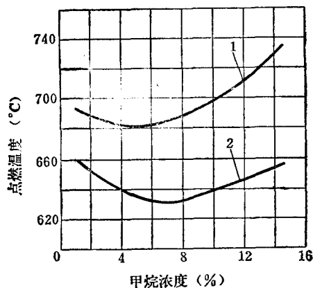
图 3-1-4 不同容器点燃温度与浓度的关系 曲线1—容器的容积48升；曲线2—容器的容积440升
