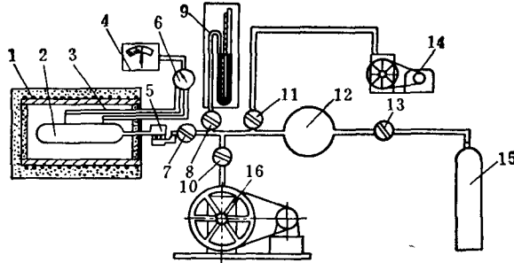
图 3-1-1 自燃温度试验装置
