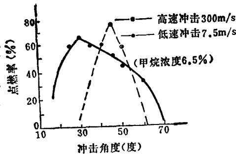
图 3-1-2 冲击角度与点燃或燃率的关系
