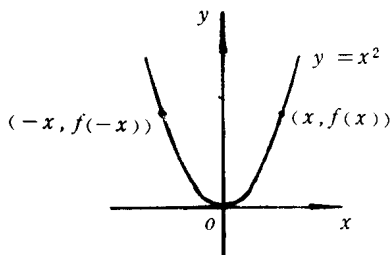
图 1.6 对称于 y 轴
