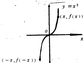
图 1.7 对称于原点
