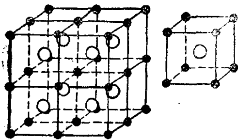
●Cs + ○Cl -
