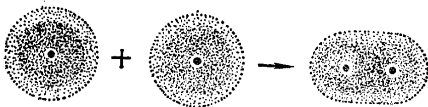
图 1-3 氢分子的形成
