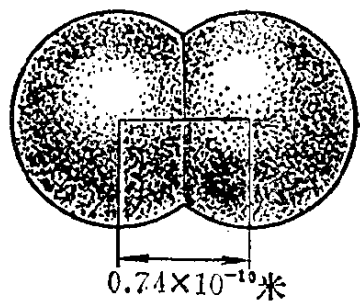
图 1-4 H-H 键的键长
