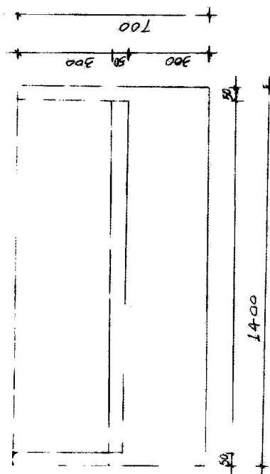
室外休息椅平面图: 1:10 (mm)
