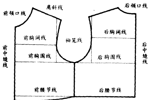
童装原型特殊部位补正表
