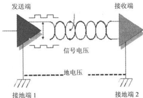
图 1.8 RS-485 的信号传输方式
