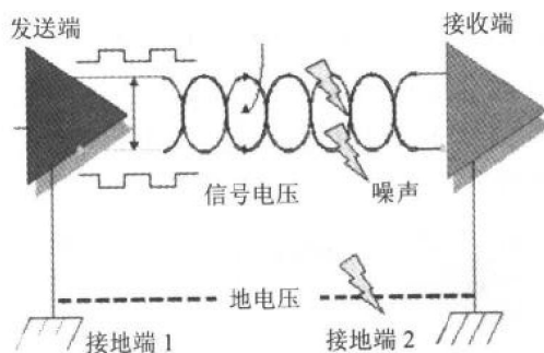
图 1.9 RS-485 传输受干扰时的情形
