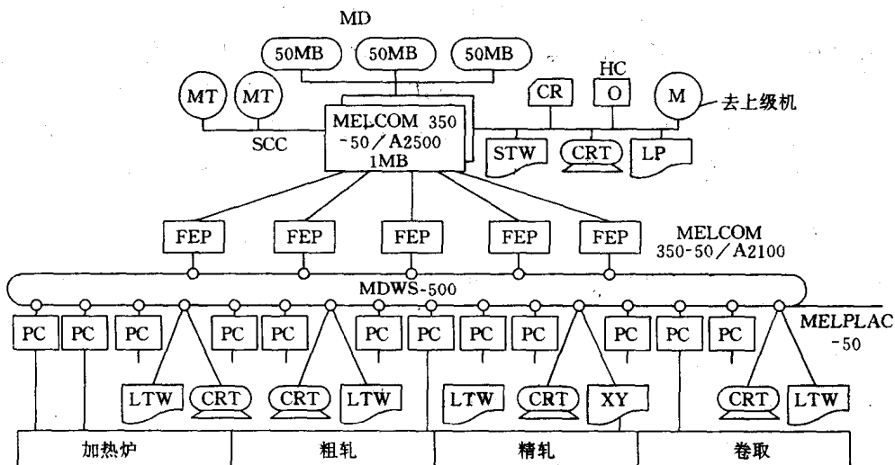
图 1.3 带钢热连轧机集散型控制系统
