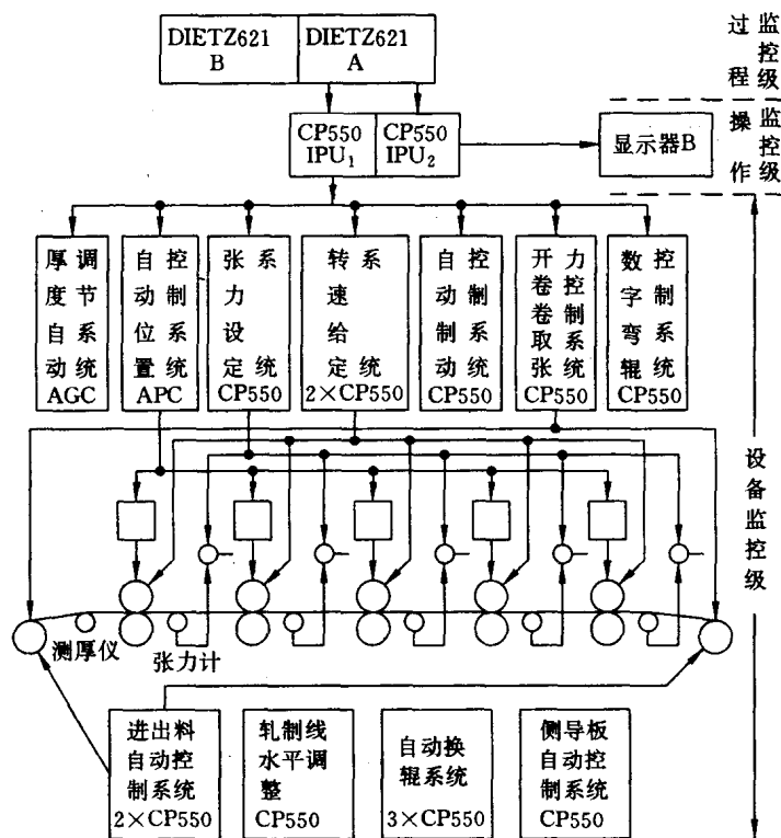
图 1.2 五机架冷连轧机控制系统
