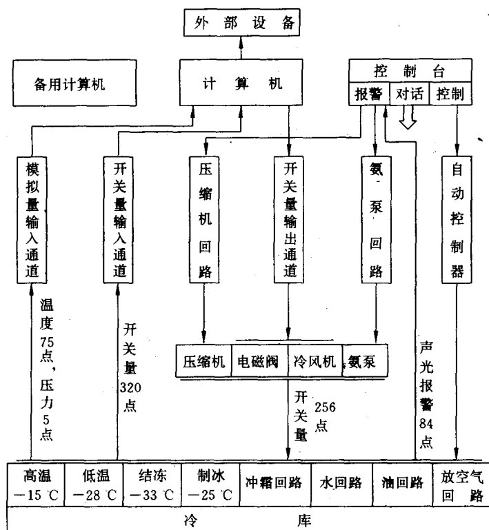
图 1.1 制冷过程计算机控制系统
