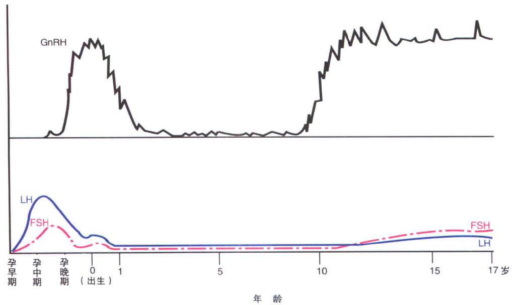
图 3-2 不同年龄阶段 GnRH 及 FSH、LH 分泌示意图
