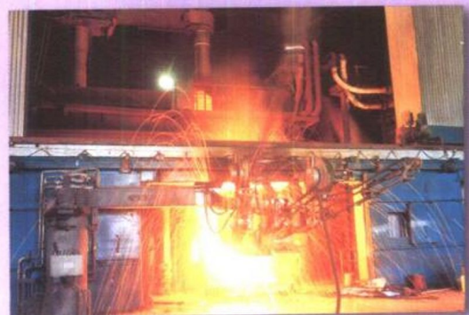
从德国引进的100t超高功率直流电炉
