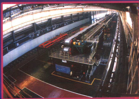
冷轧厂不锈钢冷热混合退火酸洗线
