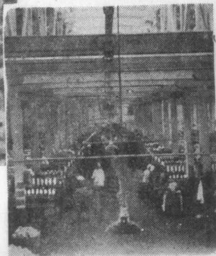
这是从創建到1952年燕湖紡織厂細紗車間的內景，仅有二万三千个左右紗錠。
