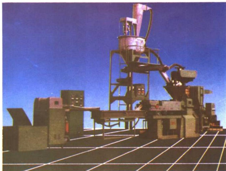
S Z J 80系列塑料造粒机组
