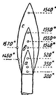
圖 3 煤氣燈火焰中的溫度分佈。
