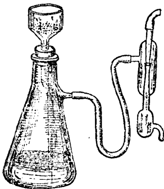
圖 19 用布氏漏斗過濾。
