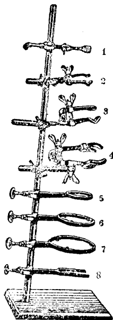
圖 12 鐵架和附件：
