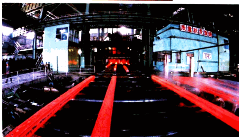
四机四流方坯连铸机
