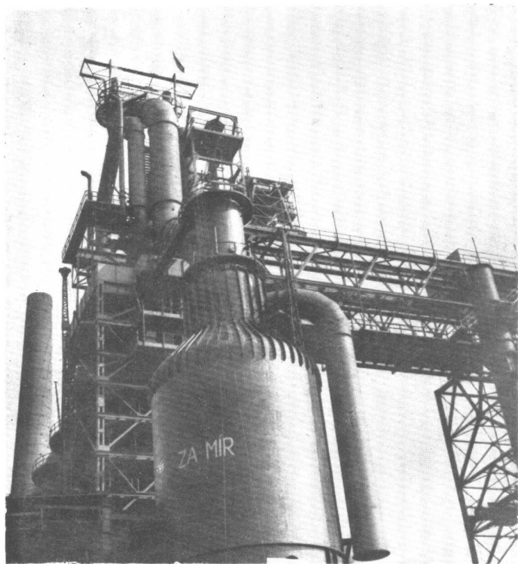
特尔息涅茨城的第六座熔鉄爐——“五一熔鉄爐”。
