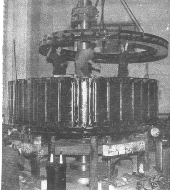
科斯托納水电站的發電機正在安裝中。
