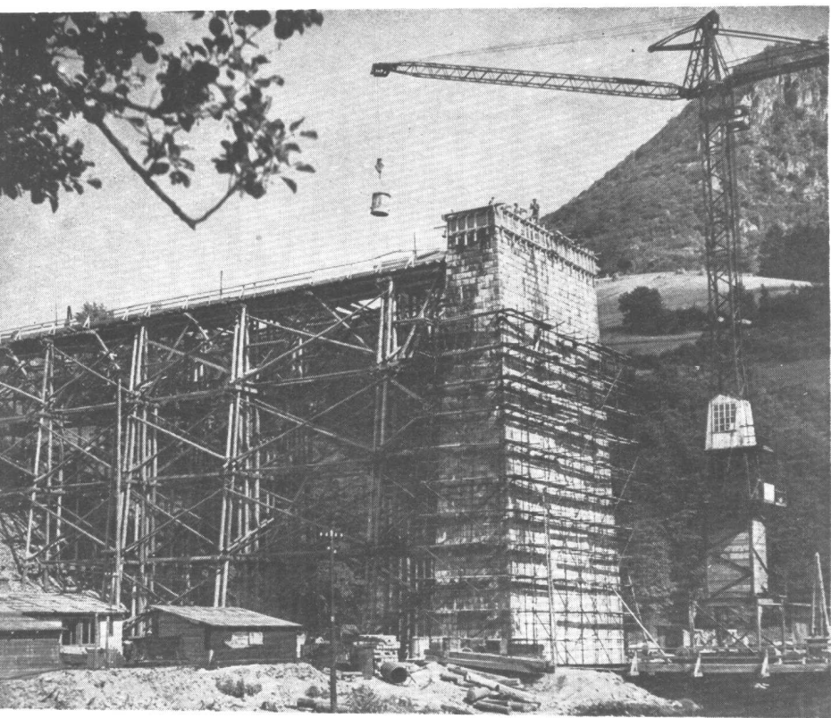
捷克斯洛伐克的最高建设工程——斯洛伐克“友谊大道”上的高架桥。
