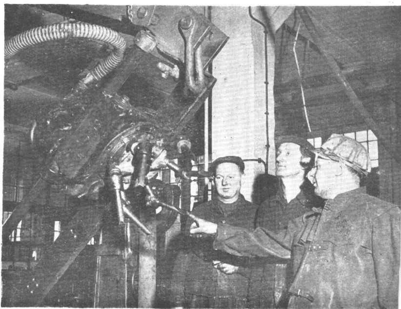
在“勝利的二月礦井”內裝置了捷克斯洛伐克的采煤聯合機“烏諾那克”。
